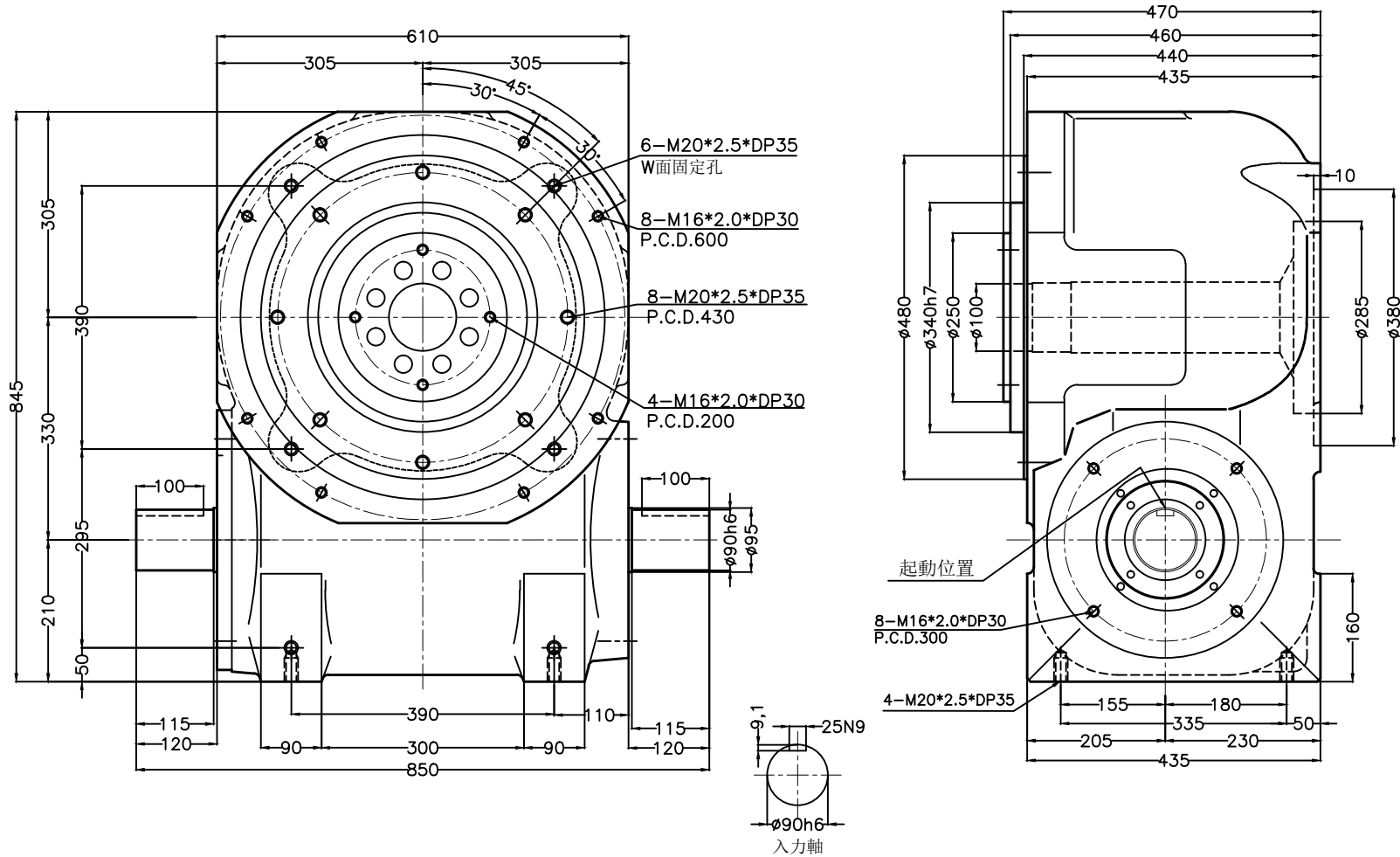
外觀圖 RU330DA
